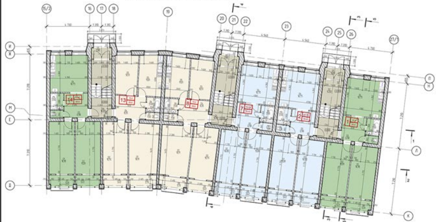
План первого этажа на отметке +0,000 (1:100)
